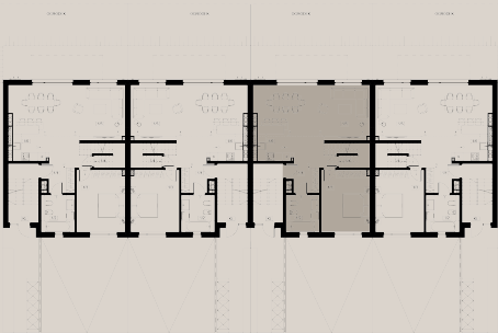
RZUT PARTERU W BUDYNKU C
