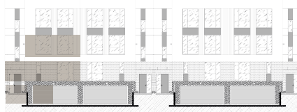
WIDOK ELEWACJI FRONTOWEJ W BUDYNKU D
