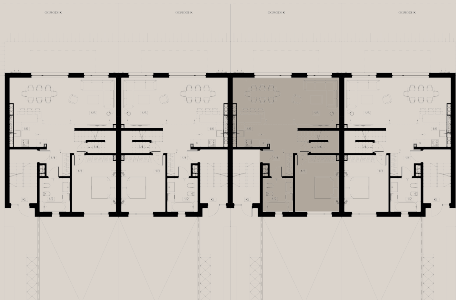
RZUT PARTERU W BUDYNKU D
