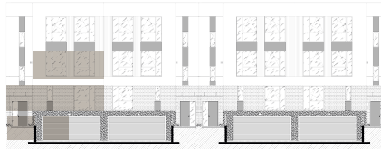
WIDOK ELEWACJI FRONTOWEJ W BUDYNKU A
