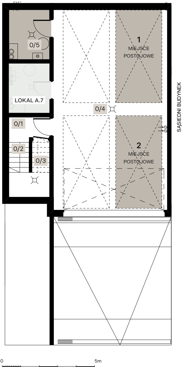
KONDYGNACJA I - PODZIEMNA
